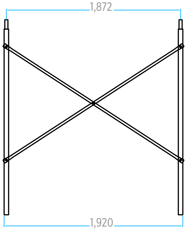
CRUCETA 2.30
